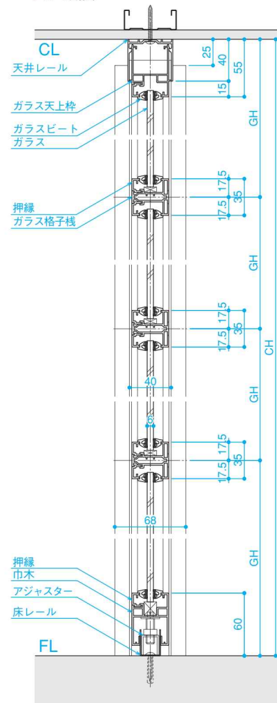
■C-C断面
