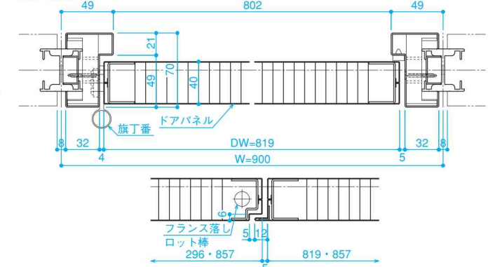
ハイトタイプ開き戸 ■C-C断面
