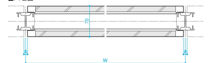
■F-F断面
