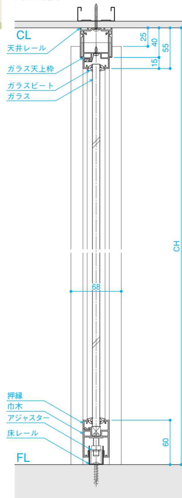
■D-D断面
