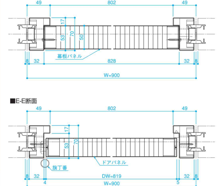
ランマ幕板タイプ開き戸 ■D-D断面
