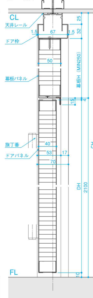
ランマ幕板タイプ開き戸 ■B-B断面
