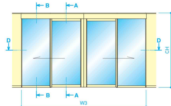
ガラス引き戸 (引分け)
