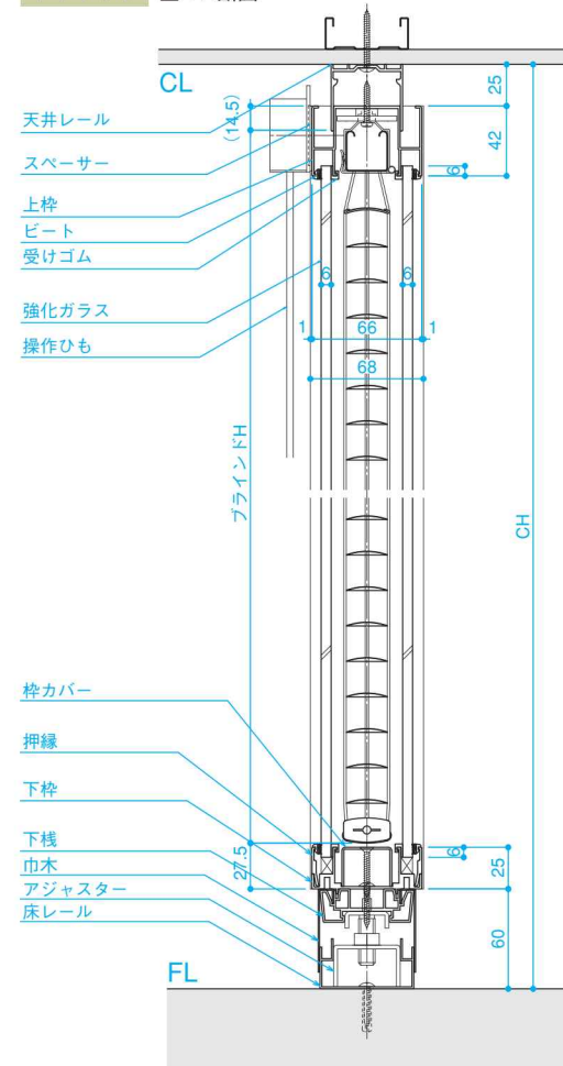
■A-A断面
