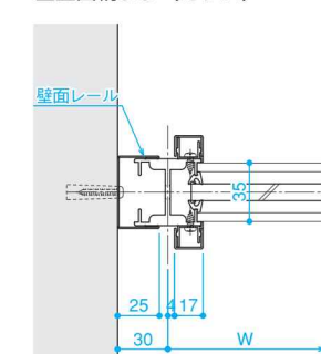
■壁面納まり (ガラス)
