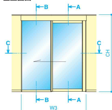
ガラス引き戸 (片引き)
