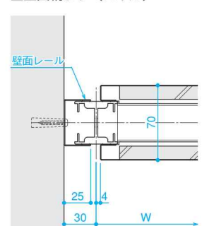
■壁面納まり (パネル)
