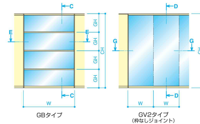
■製品寸法
