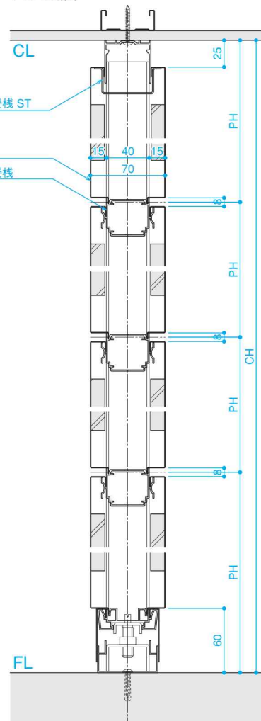
■B-B断面
