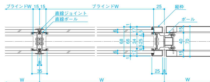
■B-B断面
