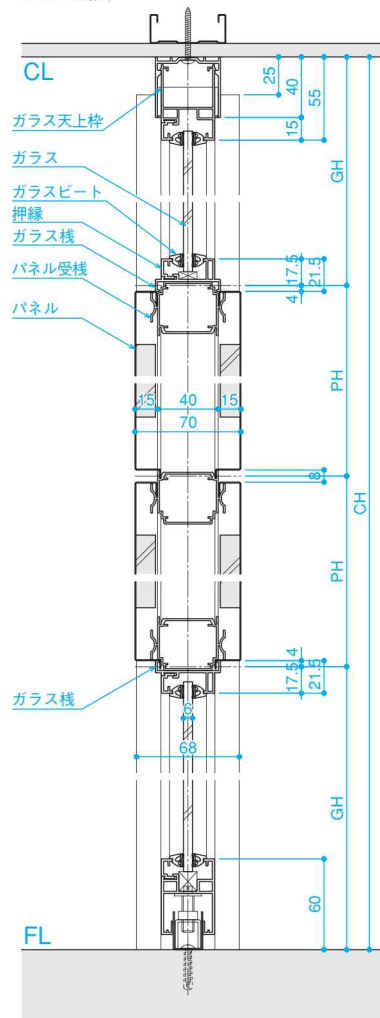
■A-A断面
