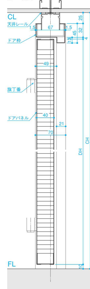
ハイトタイプ開き戸 ■A-A断面
