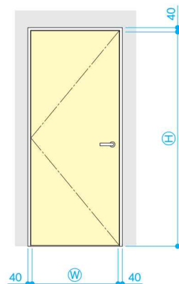
■立面図
