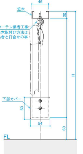
SB-AP タイプ (カーテン仕様)
