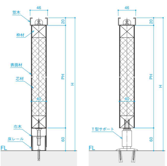
断面図 S=1/6
