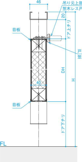
SB-GPR タイプ (メラミンSドア仕様)
