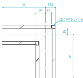
Lコーナー 全面ガラス納まり (二重ガラス)
