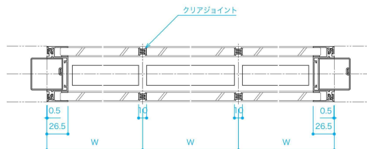
■O-O断面
