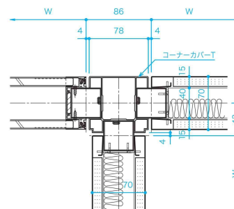
Tコーナー コーナークバー納まり
