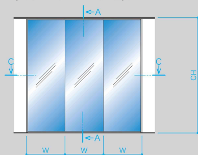
GV2タイプ (二重ガラス)
