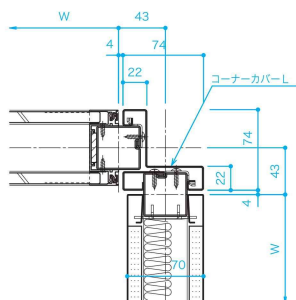
Lコーナー コーナークバー納まりA
