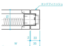
エンドフィニッシュ納まり
