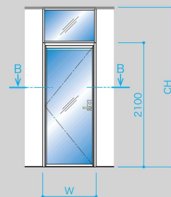
GOD-3タイプ (ランマガラス片開き戸)
