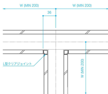
Tコーナー 全面ガラス納まり (二重ガラス)
