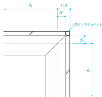
Lコーナー 全面ガラス納まり (片寄せガラス)
