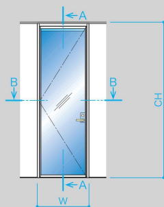
VOD-3タイプ (ハイトタイプ片開き戸)
