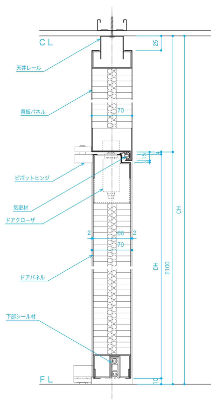
MOD-3タイプ (ランマ幕板タイプ片開き戸)
