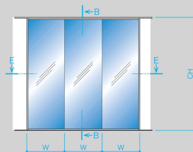
GV2タイプ (片寄せガラス)
