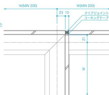
Tコーナー 全面ガラス納まり (片寄せガラス)
