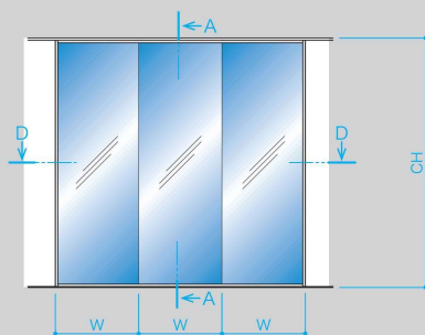
GV2タイプ (スマートインナーボール仕様)
