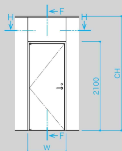
POD-3タイプ (片開き戸)
