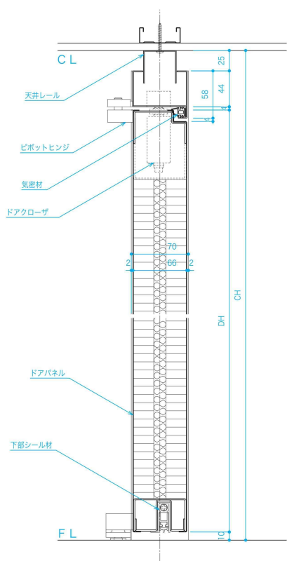
VOD-3タイプ (ハイトタイプ片開き戸)
