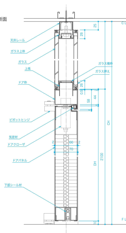
GOD-3タイプ (片開き戸)
