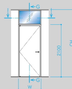
GOD-3タイプ (片開き戸)
