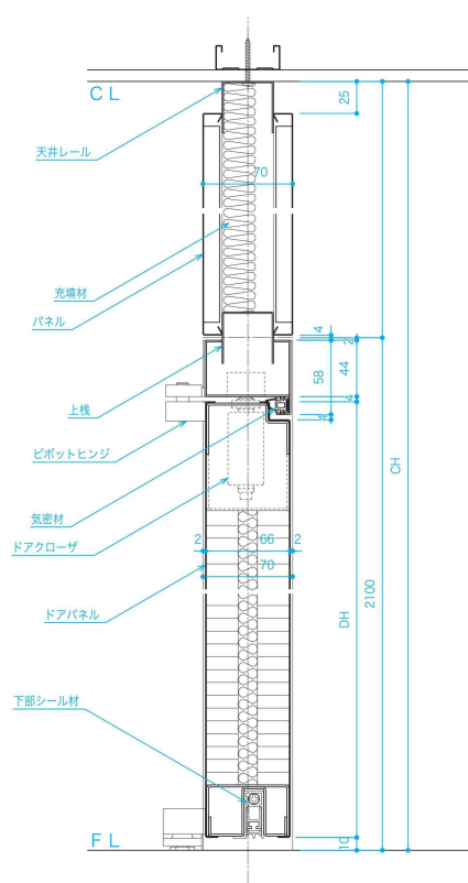
POD-3タイプ (片開き戸)
