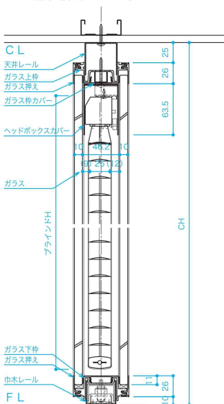
■O-O断面
