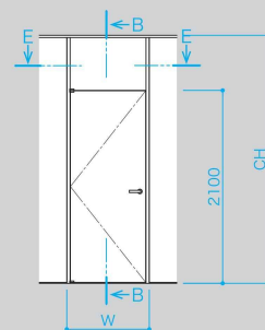
MOD-3タイプ (ランマ幕板タイプ片開き戸)
