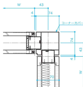
Lコーナー コーナークバー納まりB
