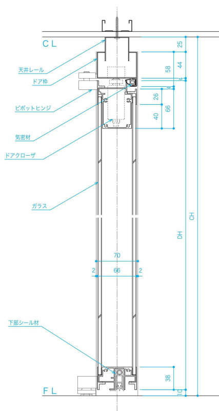
VOD-6タイプ (ハイトタイプ両開き戸)
