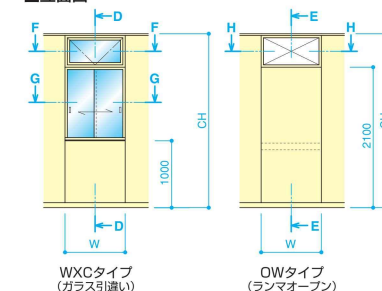
■立面図
