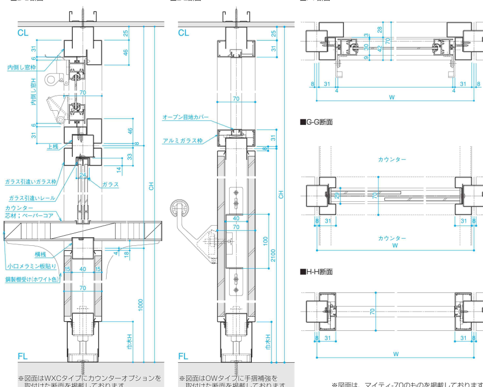
■D-D断面
