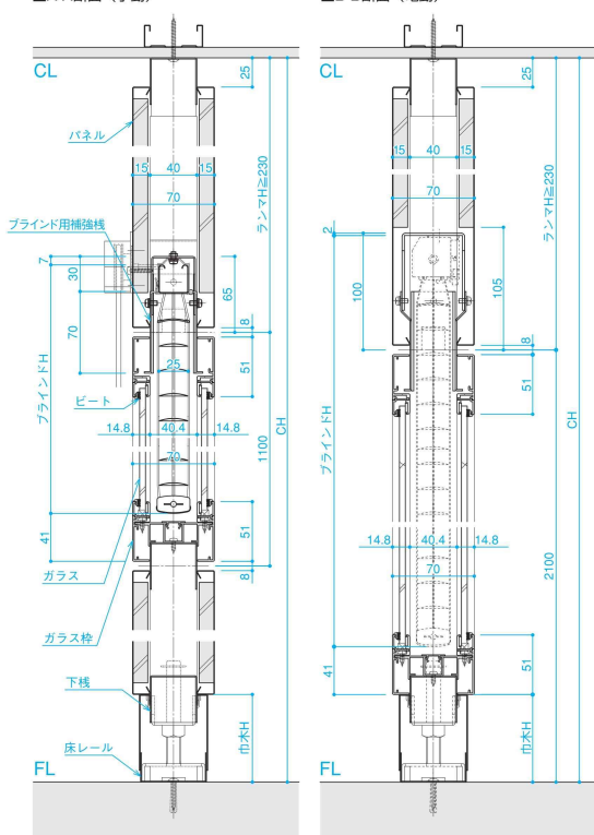
■A-A断面（手動）
