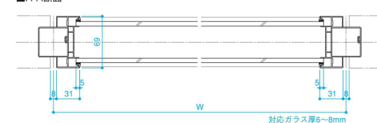
■H-H断面
