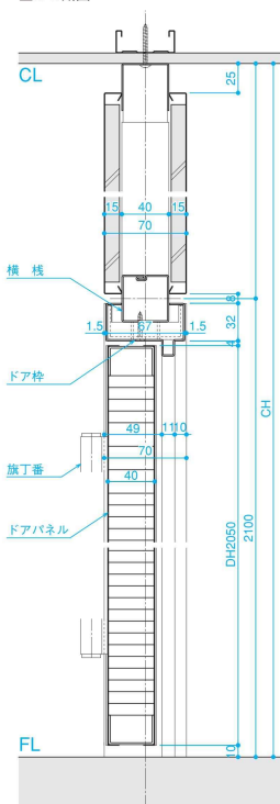
■D-D断面
