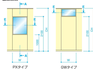
■立面図
