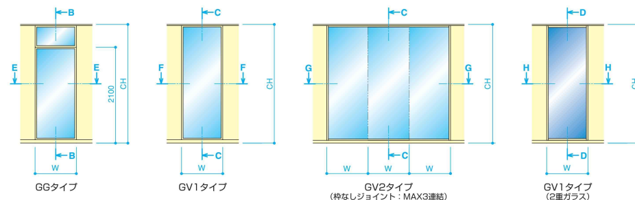
■製品寸法 (全面ガラス)
