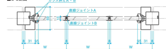
■G-G断面
