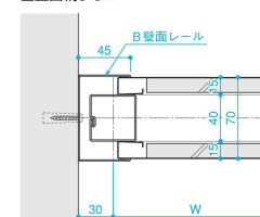
■壁面納まりB
