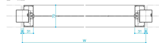
■E-E断面
