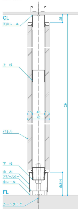
■A-A断面
