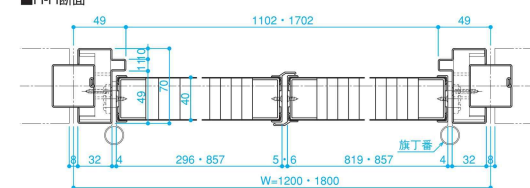
■H-H断面
