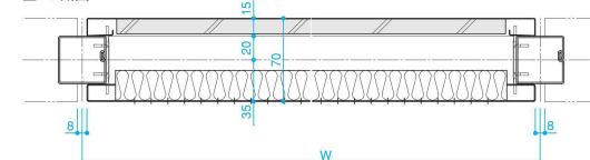
■G-G断面
