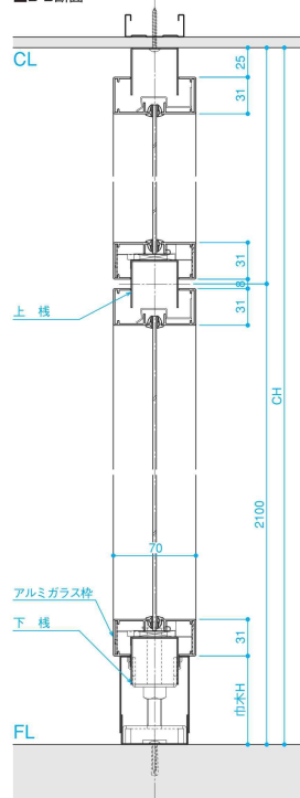
■B-B断面
