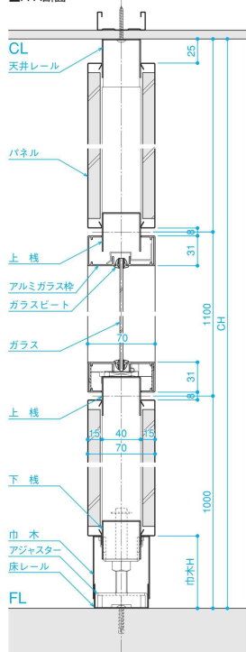
■A-A断面
