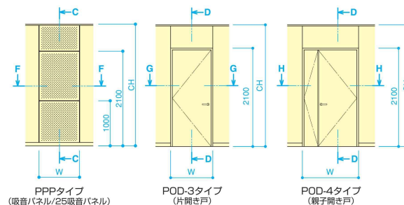
■製品寸法
