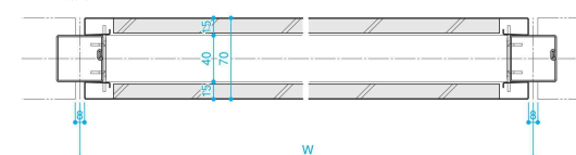
■F-F断面
