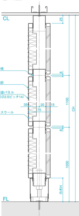
■C-C断面
