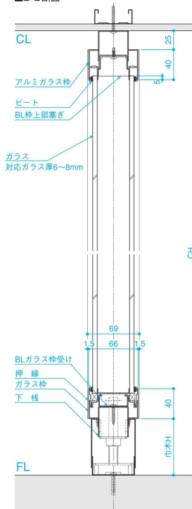
■D-D断面
