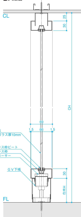
■C-C断面
