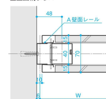
■E-E断面
