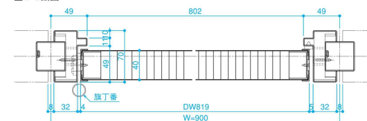
■H-H断面
